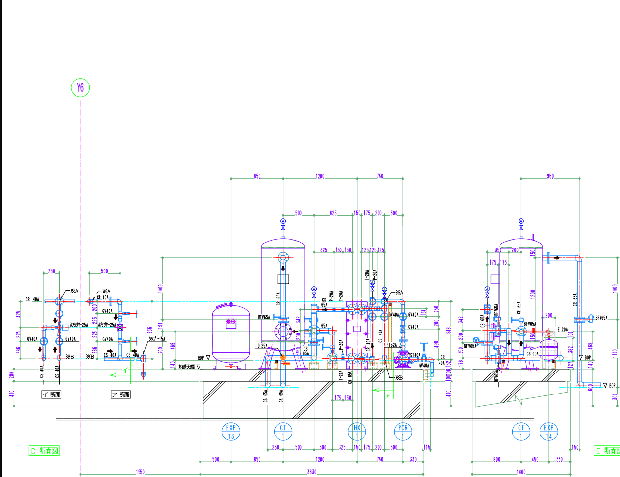
サンプル: 屋上機器廻り断面詳細図
